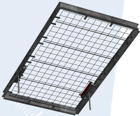
Vue de dessous grilles posées sur costière
